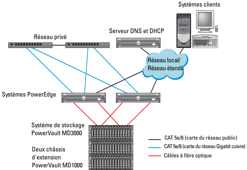
Figure 4-1. Câblage du cluster SAS et du châssis de stockage Dell PowerVault MD3000
